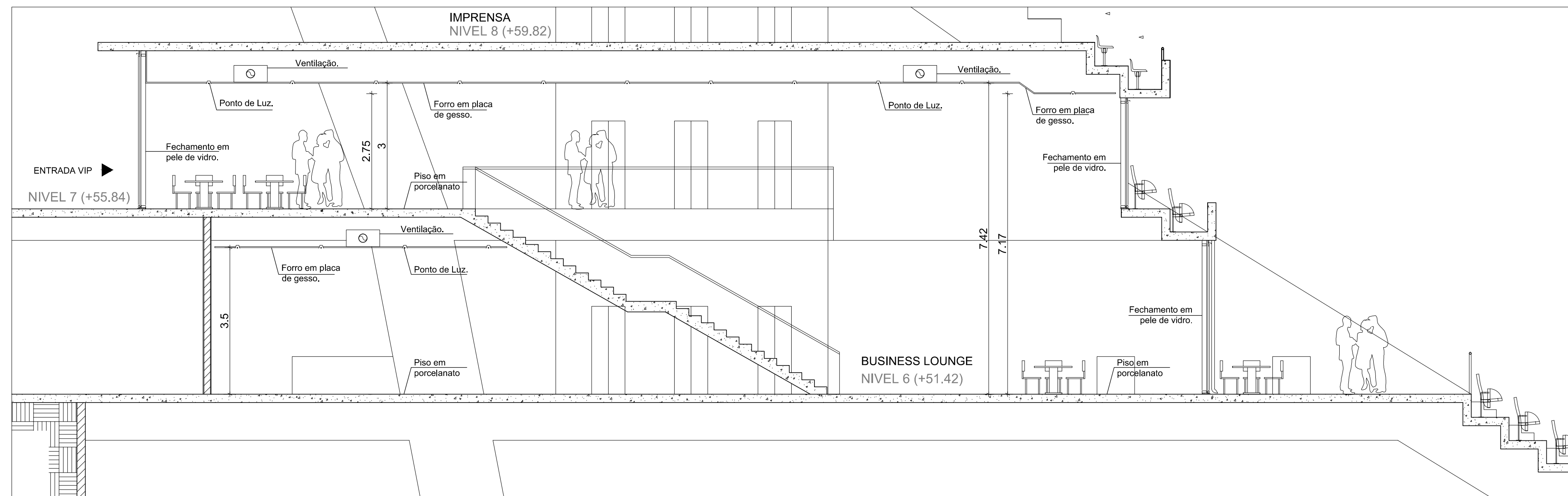
2 CORTE - BUSINESS LOUNGE ESC. 1:75
